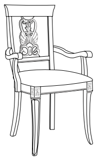
Art. 1734/C Capotavola con fondino Upholstered chair, with armrests Полукресло, облицованное 55 x 55 x 89 cm 21,67 x 21,67 x 35,07 inch nr. colli / nr. of items / количество грузовых мест: 1 m 3 : 0,34 peso netto / net weight / вес нетто: 8 kg peso lordo / gross weight / вес брутто: 12 kg
